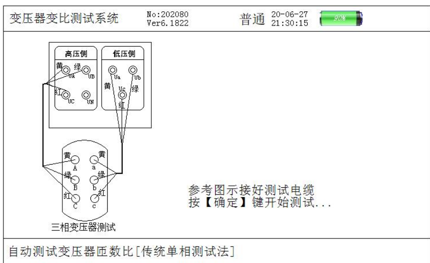
图七、三相匝数比测试接线提示屏
