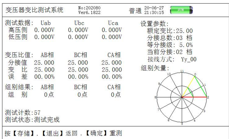
图八、三相匝数比测试结果屏
