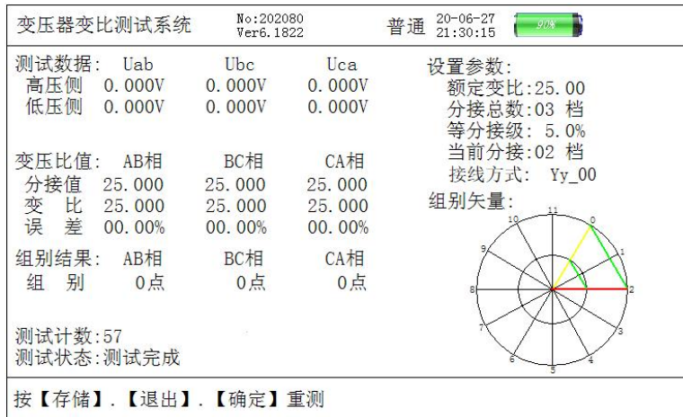
图六、三相变压比测试结果屏
