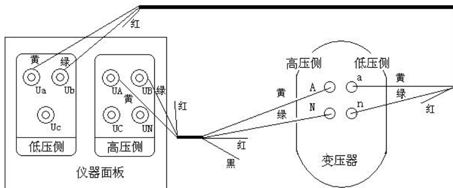
图十五、单相变压器的测试接线
