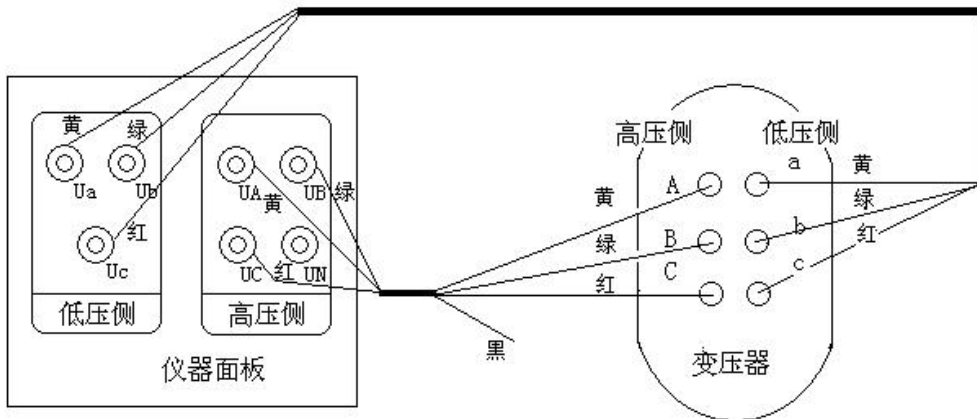
图十四、三相变压器的测试接线
