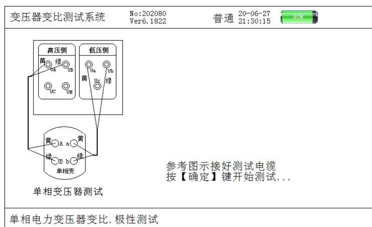
图九、单相变压器测试接线提示屏
