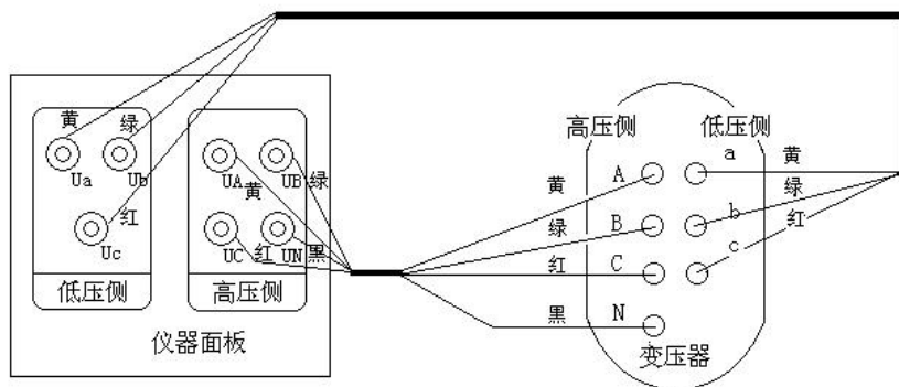
图十六、Z 型变的测试接线
