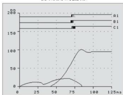
合闸测试图形
