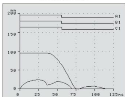
合--分闸测试图形
