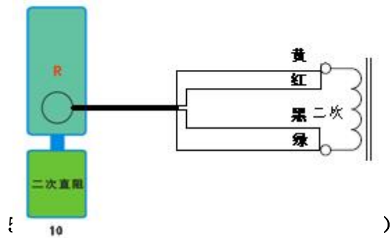
4. 接线图：图七 （二次直阻接线图）
